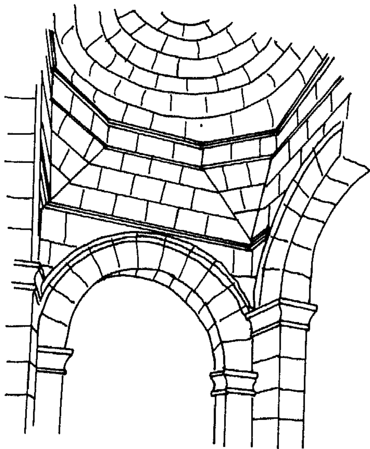
شكل (٢٥) وضع قبة التيترايبلون في اللاذقية (عن : Creswell, Fig.369)
